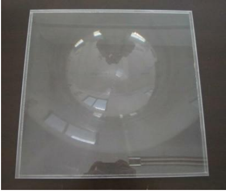
型号: HW310350 尺寸: 310*310 焦距: 350 环距: 1 厚度: 5 材质: PMMA
