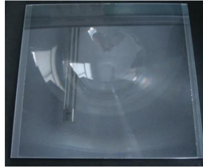
型号: HW2682501 尺寸: 268*249 焦距: 250 环距: 1 厚度: 3.75 材质: PMMA
