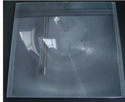
型号: HW2682651 尺寸: 268*249 焦距: 265 环距: 1 厚度: 3.75 材质: PMMA
