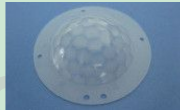
型号: 8603-4D 【048】 焦距: 17.5mm 角度: 360° 距离: 8m 尺寸: 外径 45mm 内径 32mm
